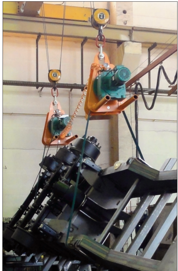
422 592: Zwei Wendegeräte WG 4, Gesamttragfähigkeit 8 t
