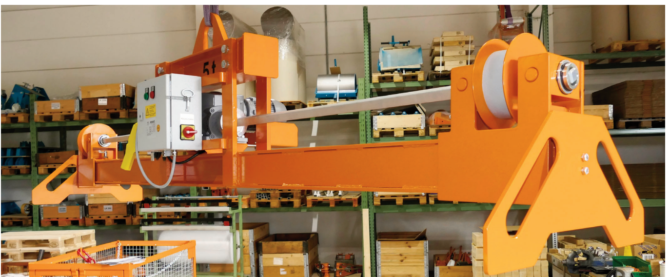
422 638 WTVE 5/3: Tragfähigkeit 5 t, Arbeitsbreite starr 3.000 mm
